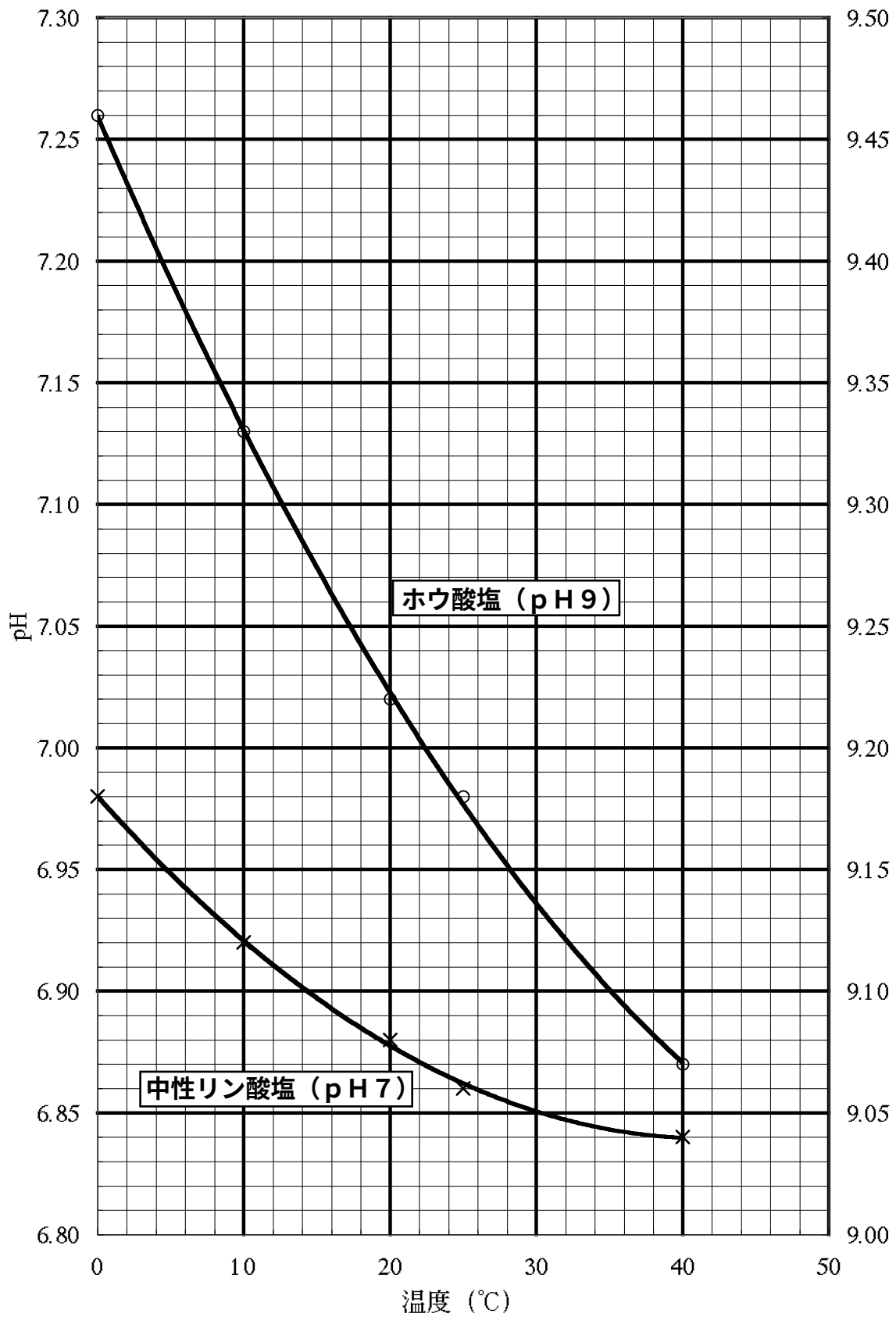
pH標準液温度特性曲線
